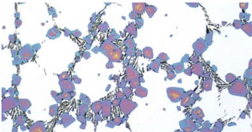
Mikrostruktur eines Nickelbasis-Lotes
