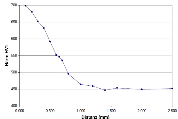
Härteverlauf durch eine einseitig gehärtete Oberfläche
